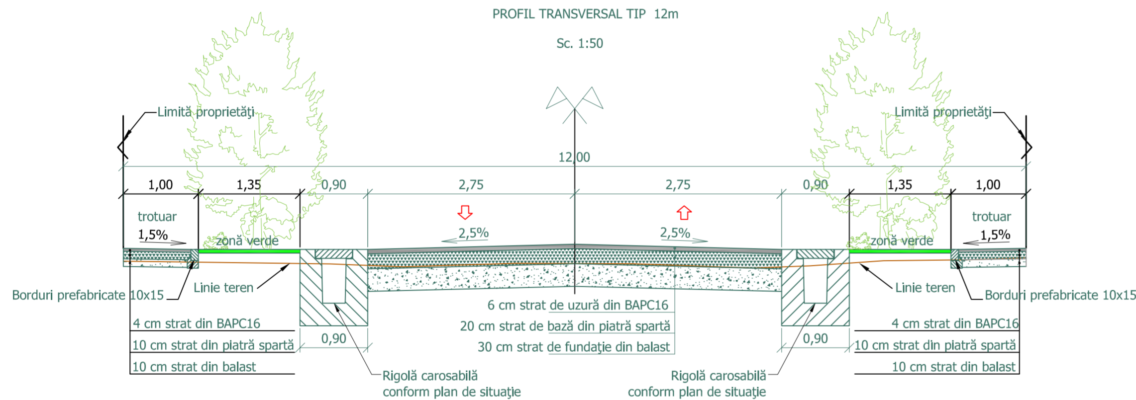
PROFIL TRANSVERSAL TIP 12m
